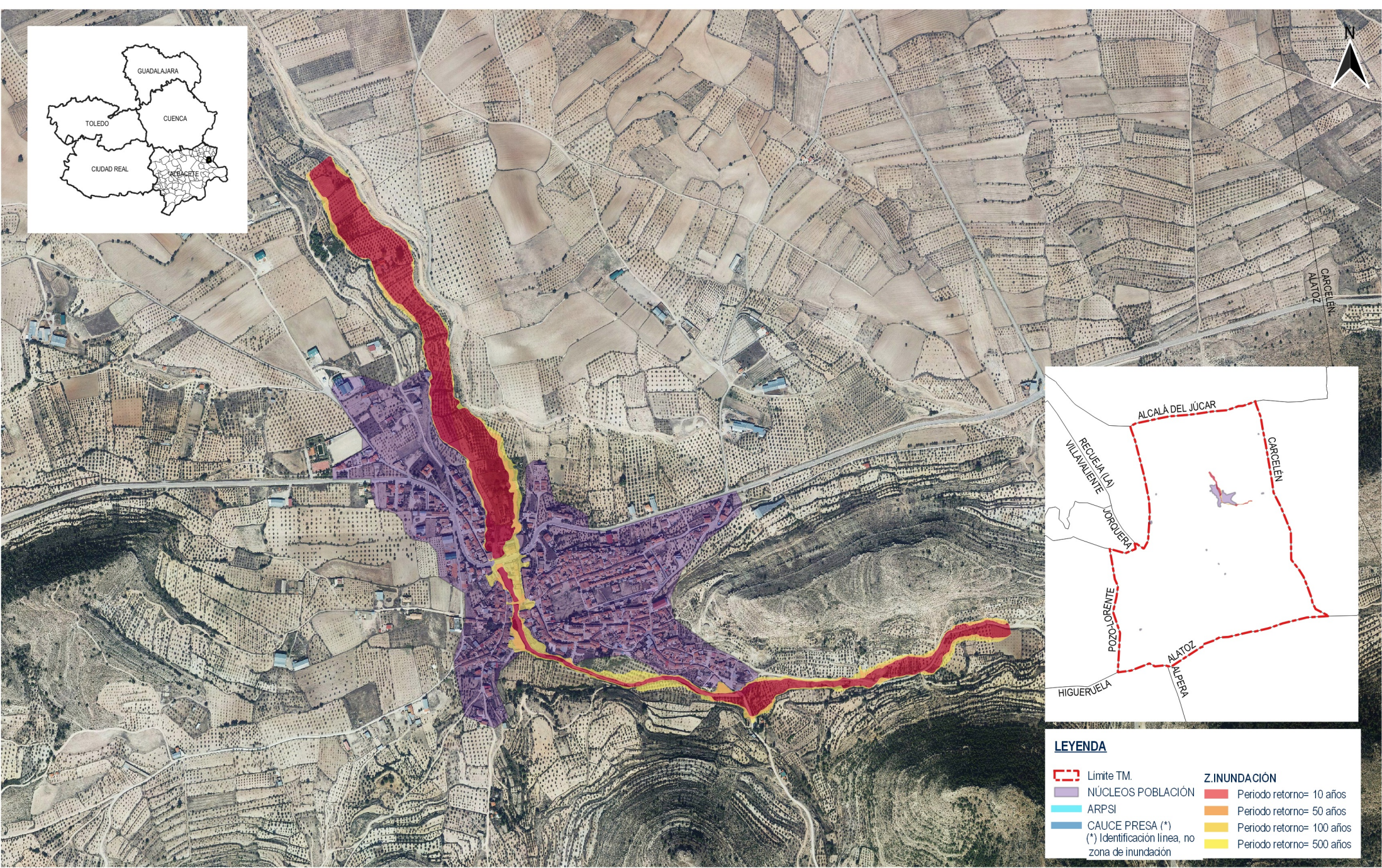
PRICAM (ED.2020) - CAP.3: ANALISIS DE RIESGO: LOCALIZACIÓN ARPSI; ZONA DE INUNDACIÓN PARA DIFERENTES PERIODOS DE RETORNO; CAUCE PRESA CON PLAN APROBADO PARA TIEMPO LLEGADA ONDA <= 2 horas.
