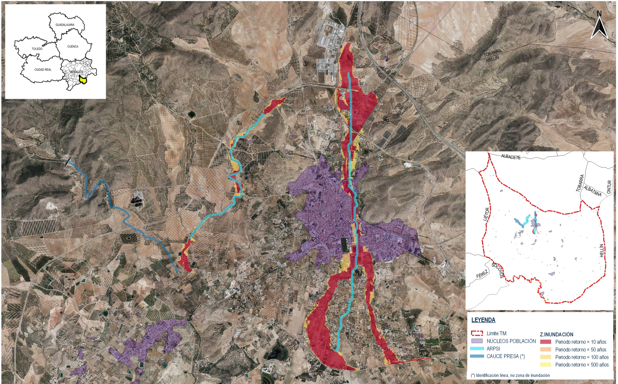
PRICAM (ED.2020) - CAP.3: ANALISIS DE RIESGO: LOCALIZACION ARPSI; ZONA DE INUNDACION PARA DIFERENTES PERIODOS DE RETORNO: CAUCE PRESA PARA TIEMPO LLEGADA ONDA <= 2 horas.
