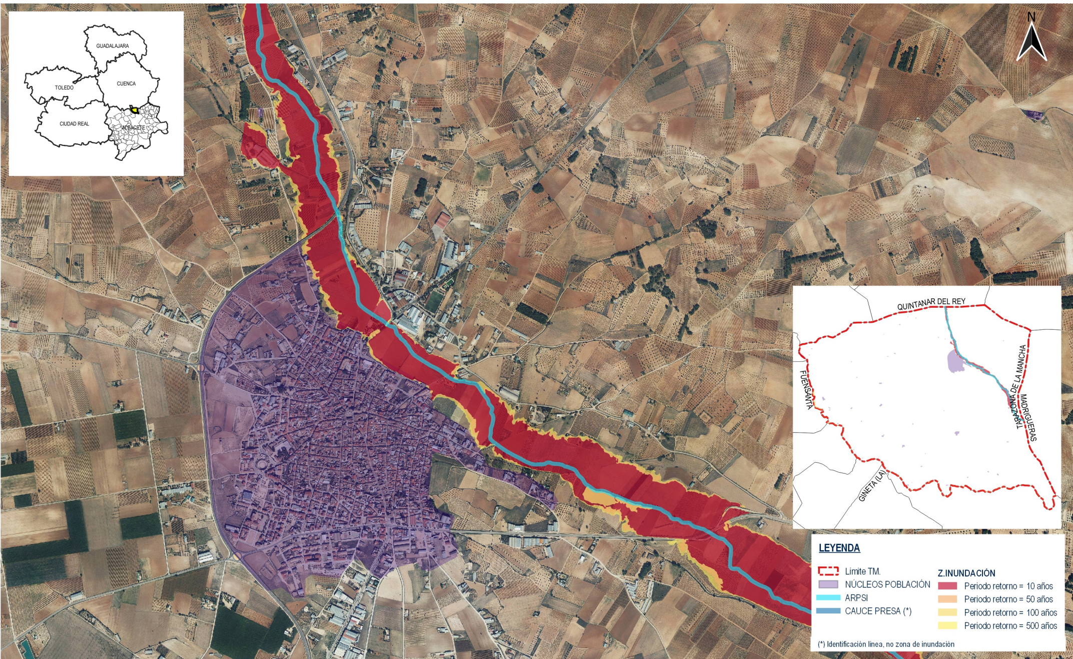
PRICAM (ED.2020) - CAP.3: ANALISIS DE RIESGO: LOCALIZACION ARPSI; ZONA DE INUNDACION PARA DIFERENTES PERIODOS DE RETORNO: CAUCE PRESA PARA TIEMPO LLEGADA ONDA <= 2 horas.
