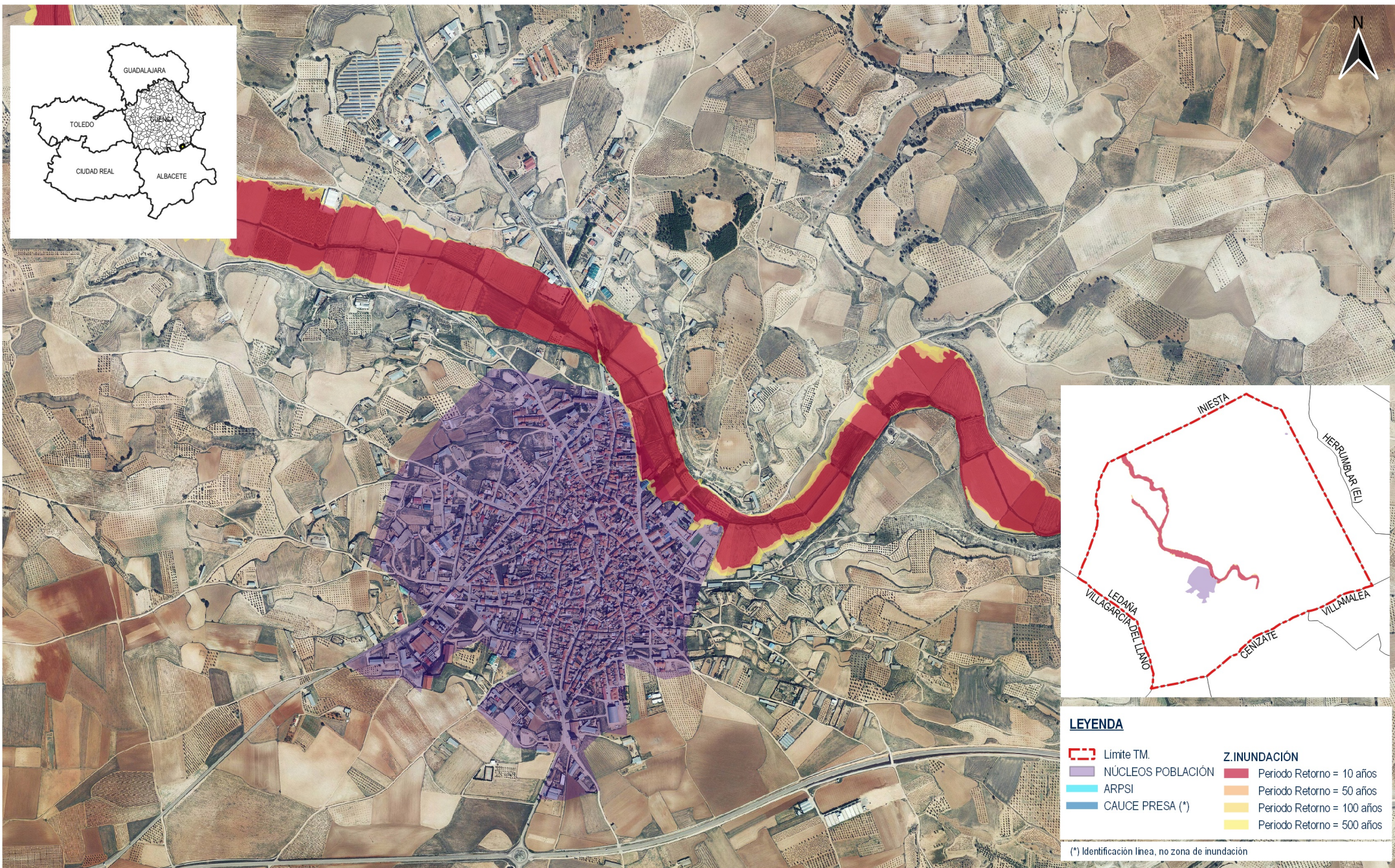
PRICAM (ED.2020) - CAP.3: ANALISIS DE RIESGO: LOCALIZACIÓN ARPSI; ZONA DE INUNDACIÓN PARA DIFERENTES PERIODOS DE RETORNO; CAUCE PRESA PARA TIEMPO LLEGADA ONDA <= 2 horas.
