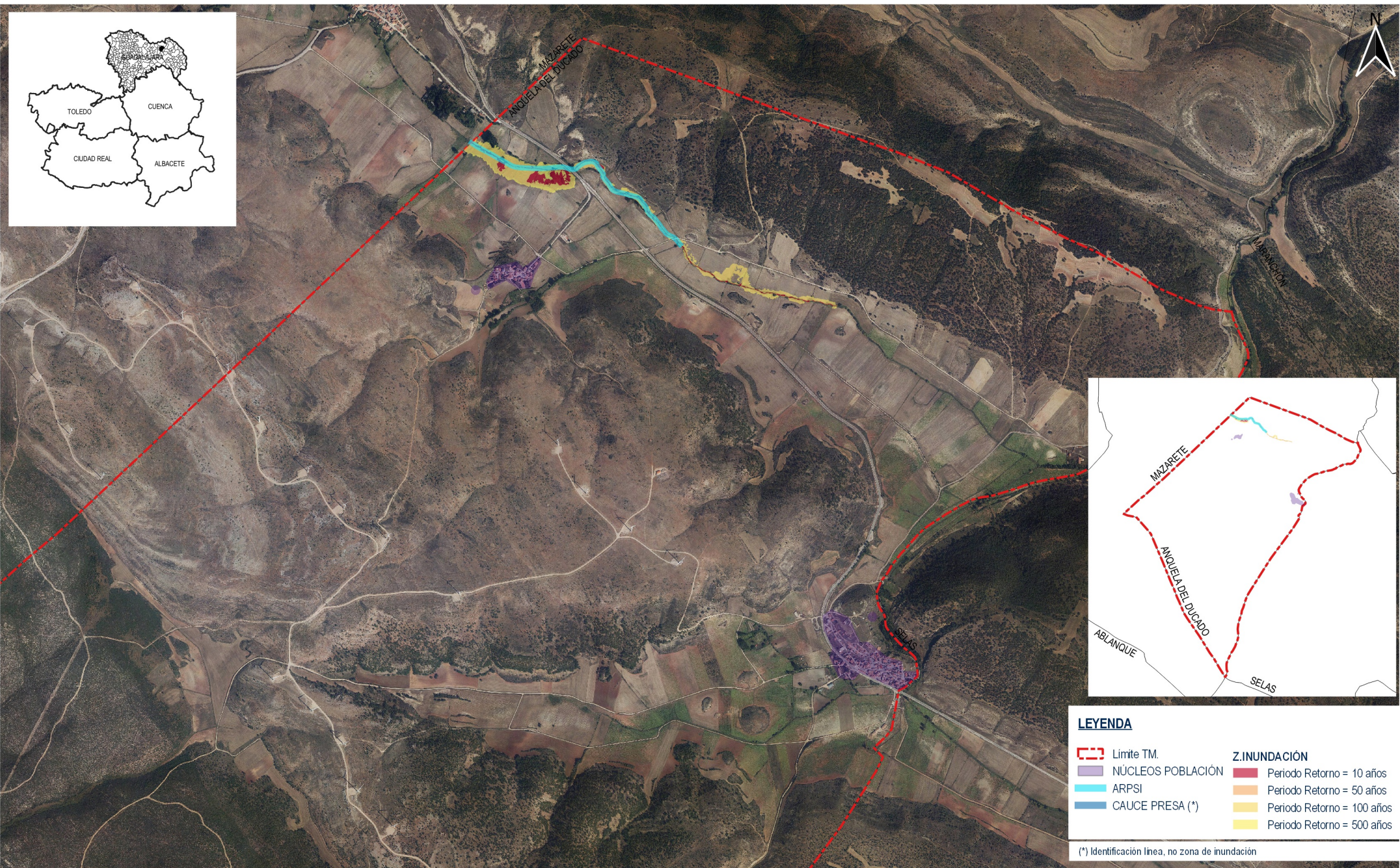
PRICAM (ED.2020) - CAP.3: ANALISIS DE RIESGO: LOCALIZACIÓN ARPSI; ZONA DE INUNDACIÓN PARA DIFERENTES PERIODOS DE RETORNO; CAUCE PRESA PARA TIEMPO LLEGADA ONDA \leq 2 horas.
